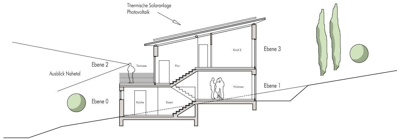
Querschnitt
